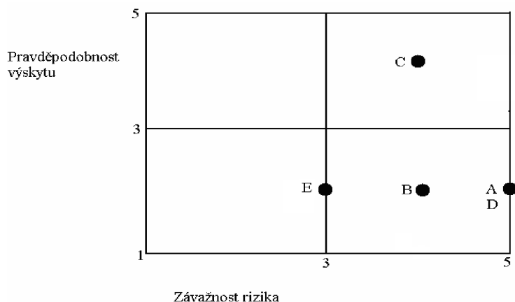
Obrázek 3 Matice rizik
