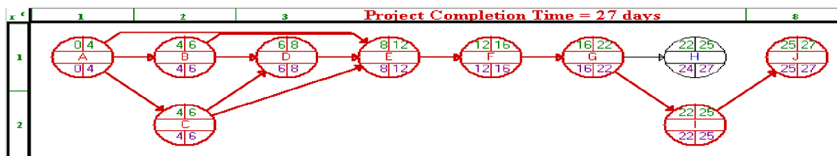
Obrázek 2 Grafické vyjádření časové analýzy se zdůrazněním kritické cesty
