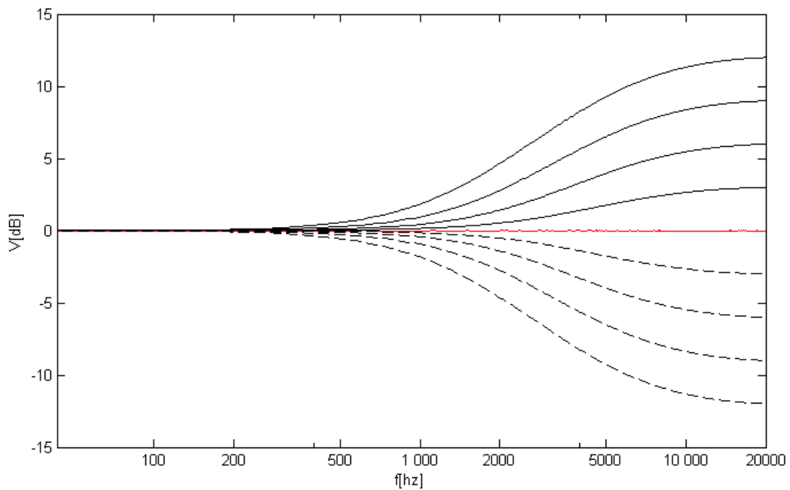
Obr. 6.3: Frekvenční odezva navrženého high-shelving filtru.
