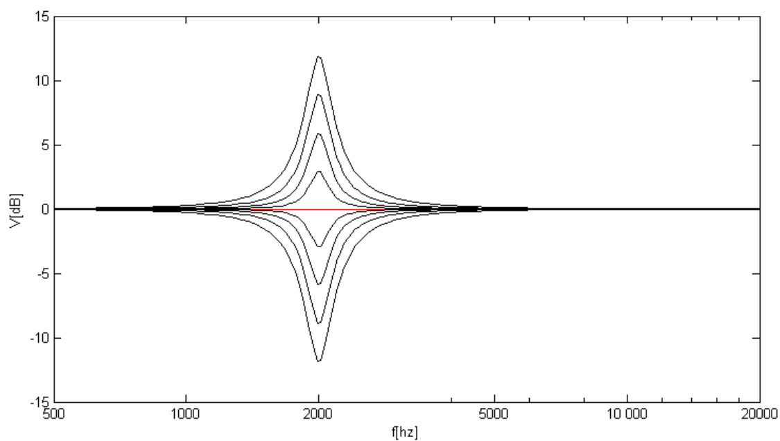
Obr. 6.6: Frekvenční odezva navrženého peak filtru pro střední frekvenci f_c=2000 [Hz] , šířku pásma f_b=200 [Hz] a útlum V = + - 3, 6, 9, 12[dB]
