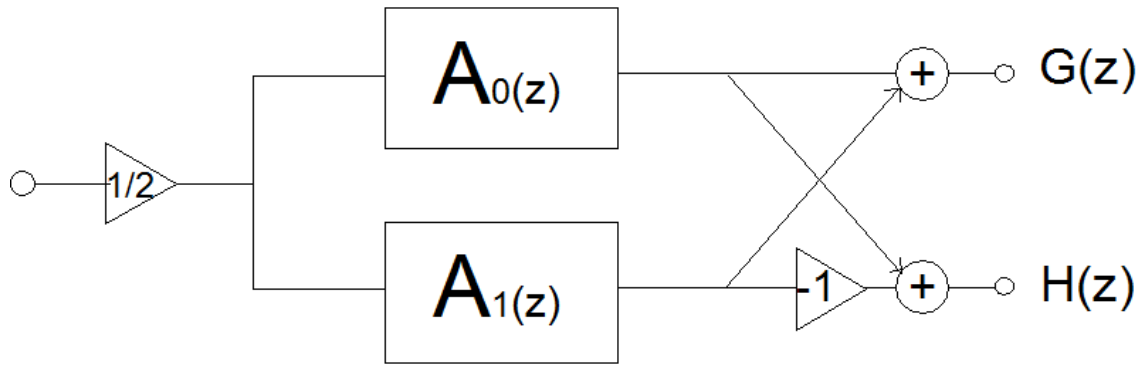
Obr. 1.3: Struktura složeného filtru realizovaného pomocí fázovacího článku.
