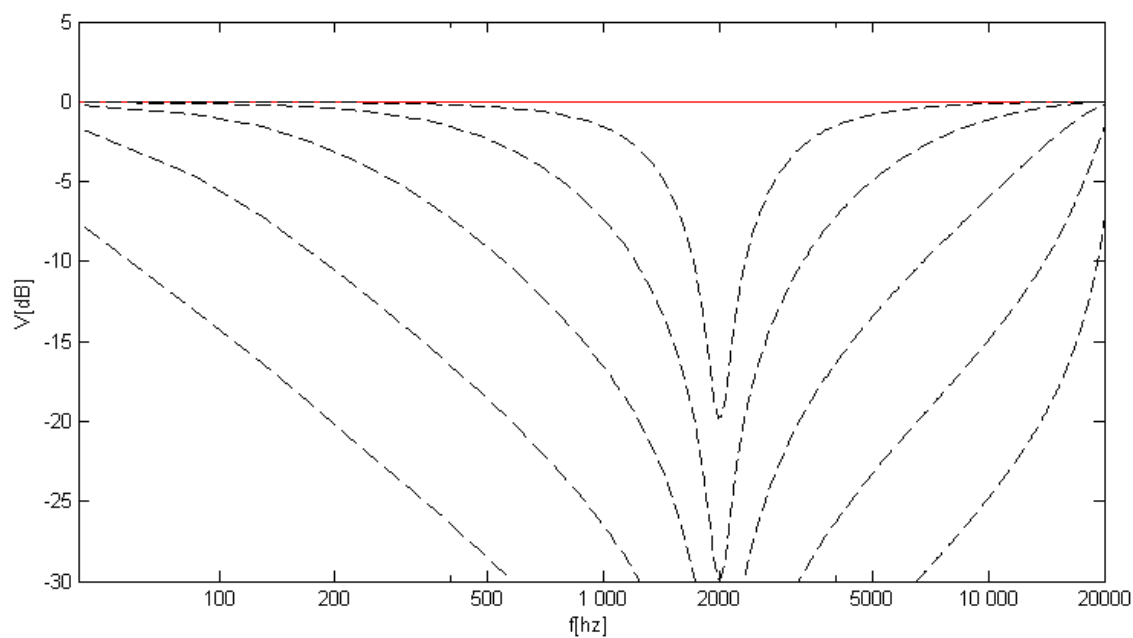
Obr. 6.7: Frekvenční odezva navrženého peak filtru pro vysoké hodnoty útlumu V=20,30,40,50,60,70 [dB]
